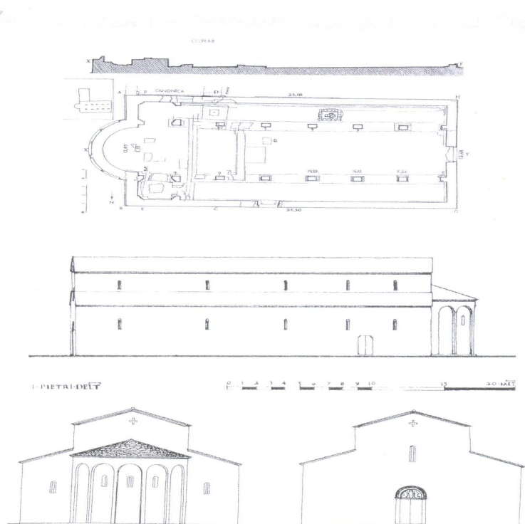
Plan, coupe et reconstitution hypothétique des façades de l'ancienne piévanie de Moriani (d'après J. Pietri)
